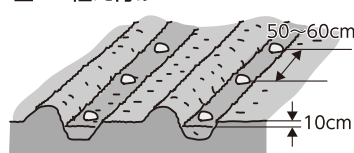
図2 植え付け
