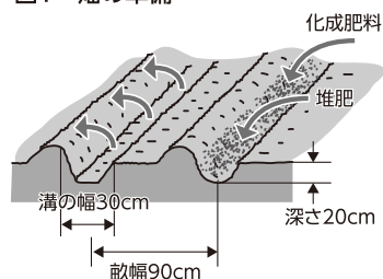
図1 畑の準備
