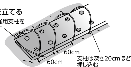
図 トンネルの作り方
